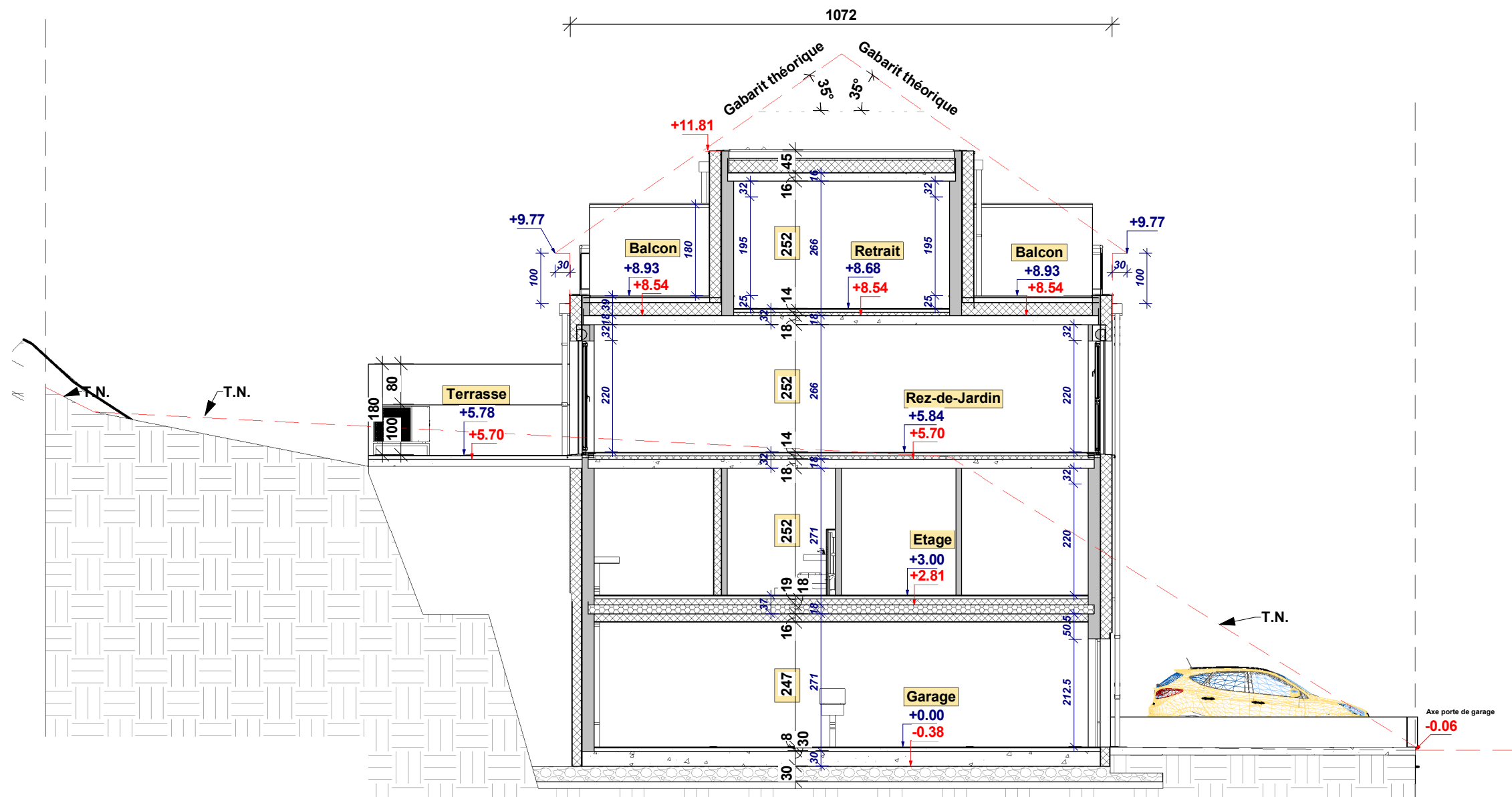
1 Coupe A-A Ech : 1 : 100
