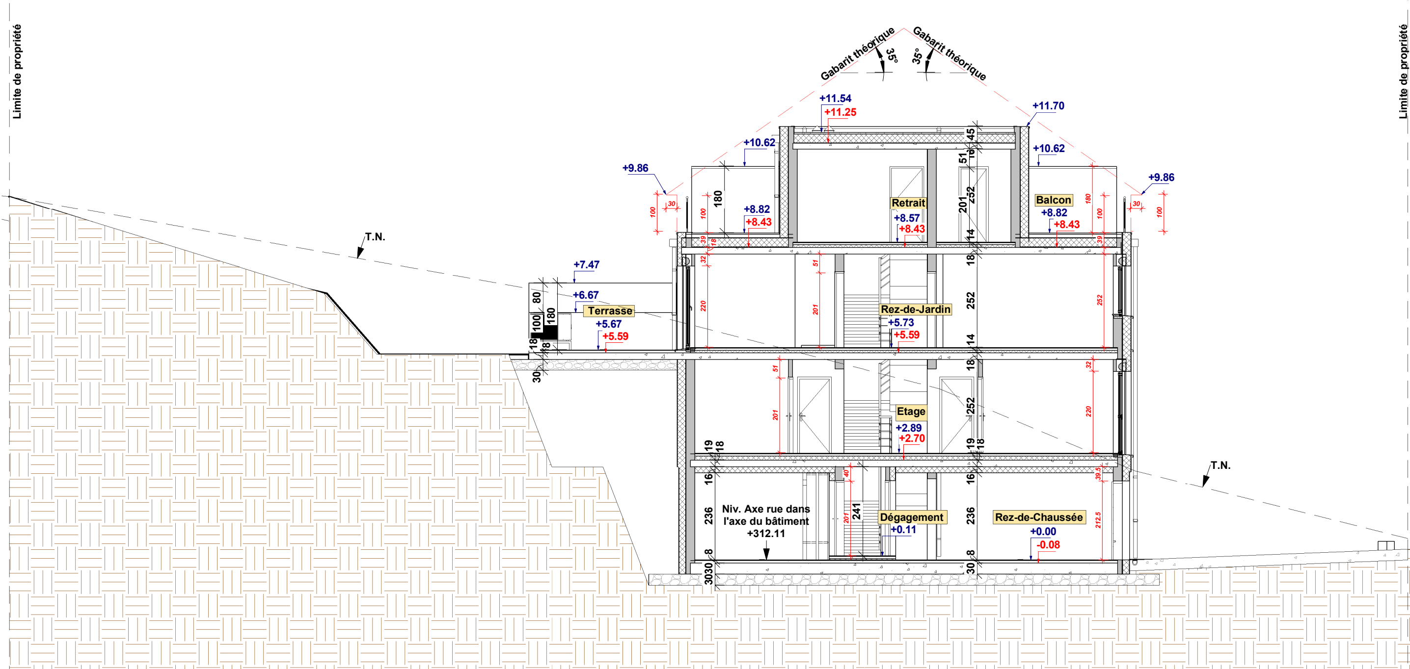
1 Coupe A-A Ech : 1 : 100
